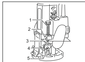
1. عمود السدادة 2. زر التغذية السريعة 3. رافعة القفل 4. المسمار السداسي 5. كتلة سدادة
