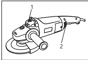
1. مخرج الهواء 2. مدخل الهواء
