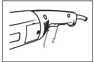
1. قفل المفتاح 2. زر الإيقاف والتشغيل
